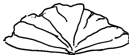
2 redondeada
