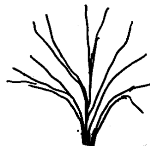
3 flabeliforme
