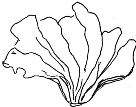
1 erecto
