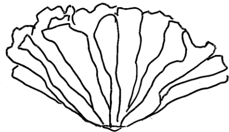
2 semierecto
