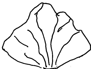
3 puntiaguda
