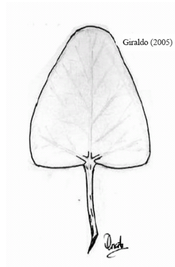
2 triangulaire
